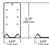
740-09 Bracket
